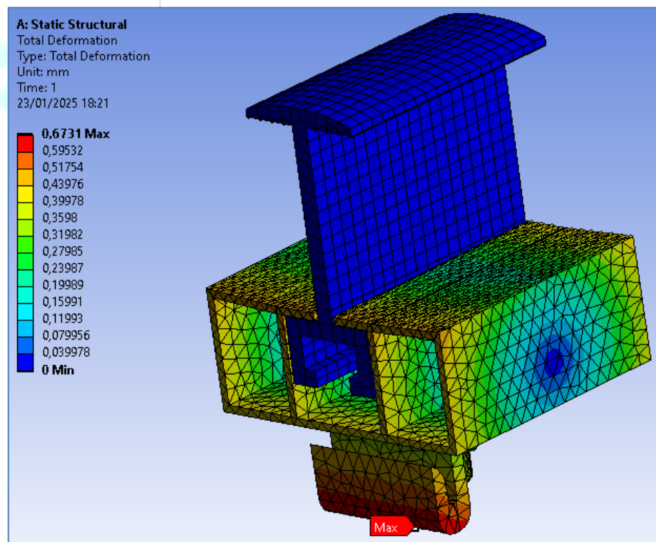
Figura 9: Resultado de deformação estática.
