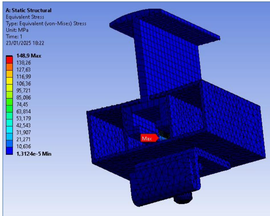
Figura 8: Resultados de tensão estática.
