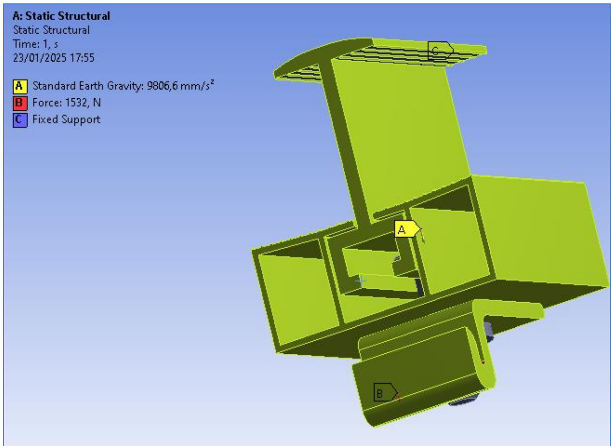
Figura 7: Ponto de aplicação de carga e fixação.
