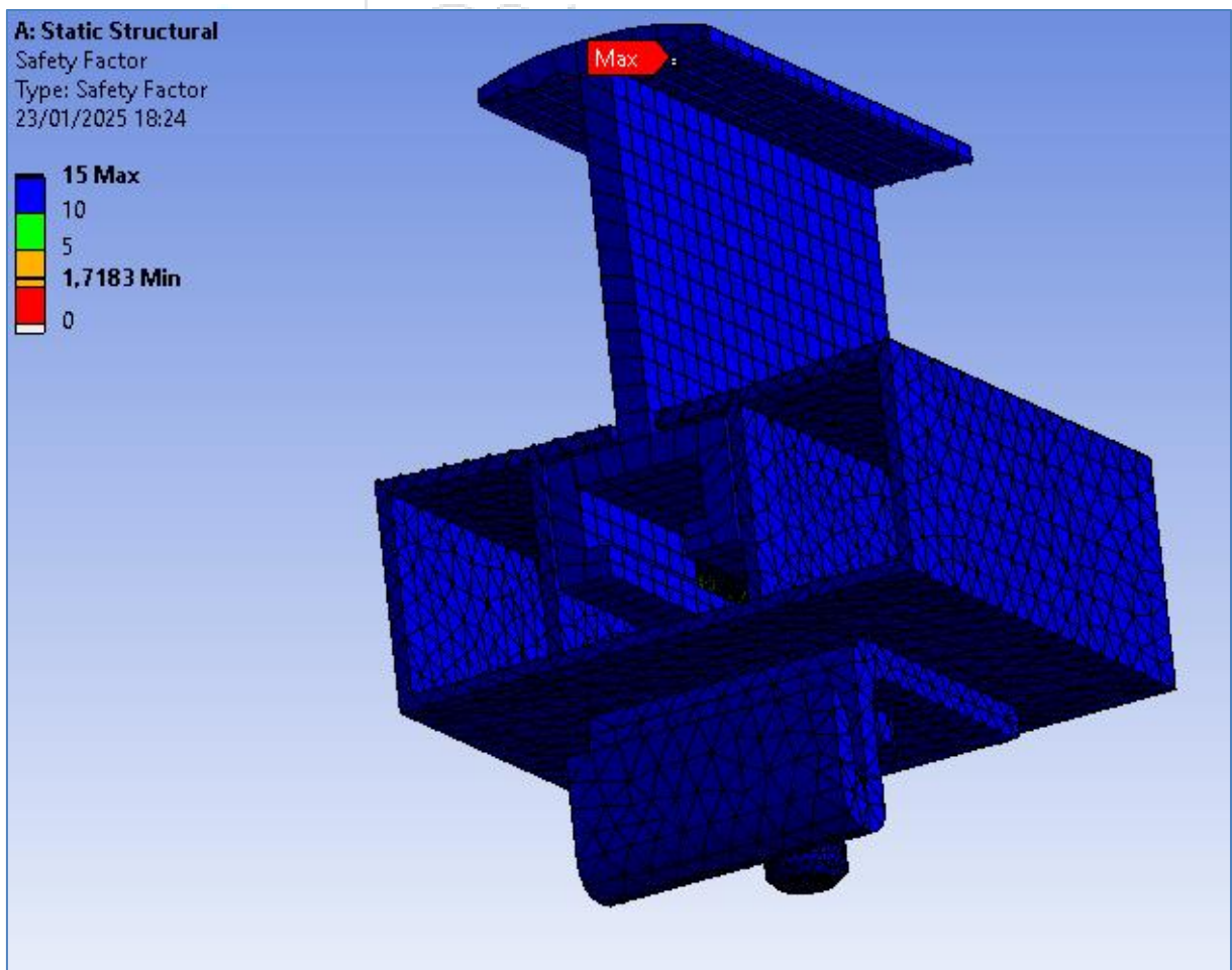
Figura 21: Resultados de fadigas.
