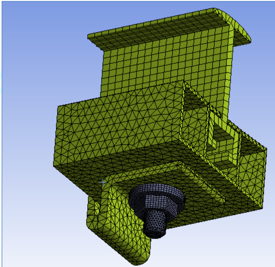
Figura 3: Malha gerada para simulação.
